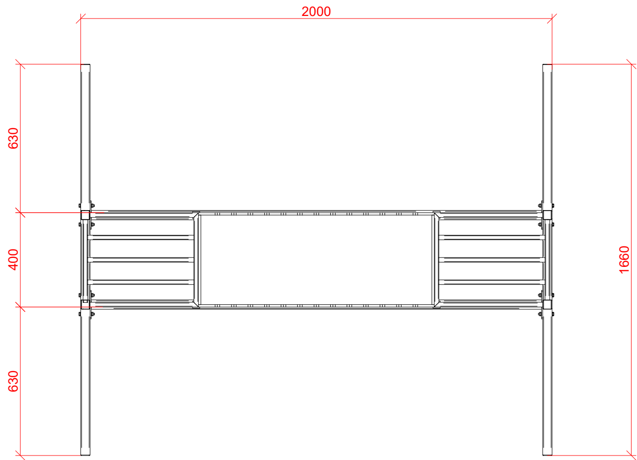
A-A (1:16)
